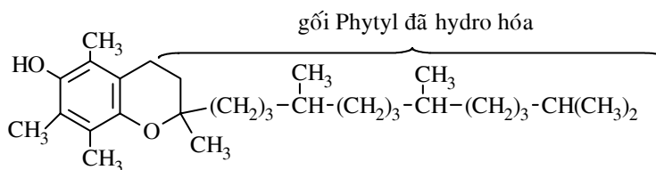
(±) \alpha -Tocopherol (thuộc nhóm vitamin E)
