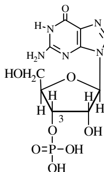
Guanylic
