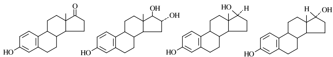
Estron
