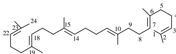
Squalen
