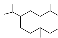
Germacran
