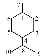
Khung p-Mentan
