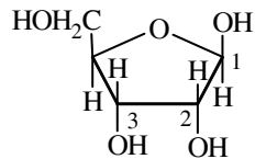
\beta -D (-)-Ribofuranose
