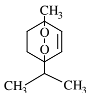
Ascaridol
