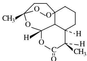
Artemisinin
