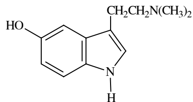
Bufotonin
