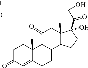
Cortison
