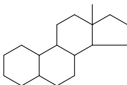
Estran
