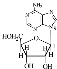
Adenosin ( Ribose + Adenin )
