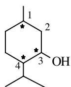
Menthol
