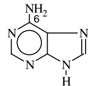
Adenin
