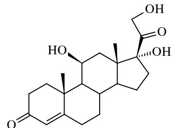
Cortisol
