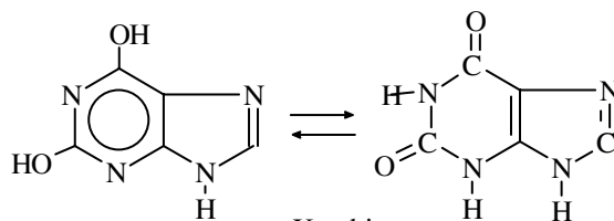
Xanthin
