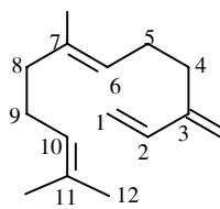
\beta -Farnesen
