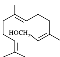
Farnesol
